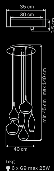
803067 CHROME smoky люстра подвесная
