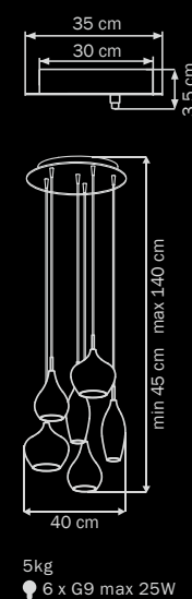
803068 CHROME olive люстра подвесная
