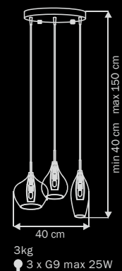
803057 CHROME smoky люстра подвесная
