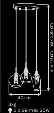
803059 CHROME plum люстра подвесная
