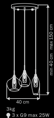
803058 CHROME olive люстра подвесная
